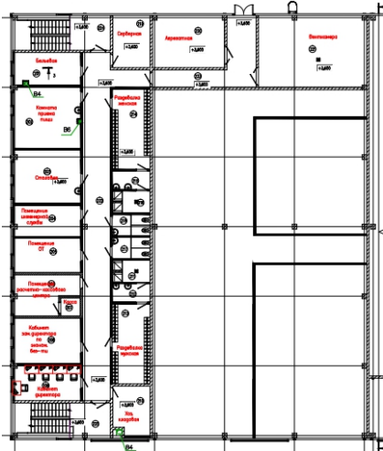
Антресоль административно-бытовой части
