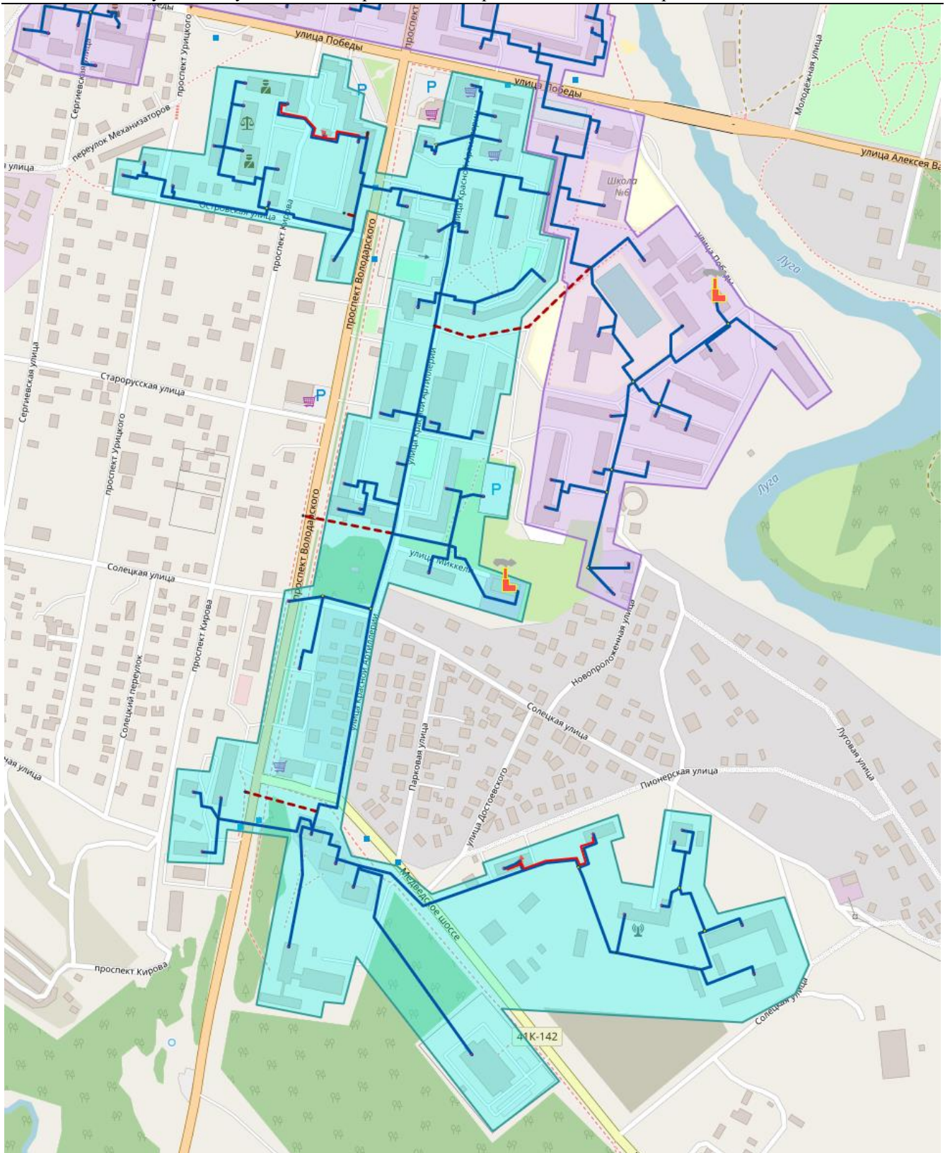
Рисунок 48 Зона действия котельной БМК-24,42, Южный-2 (ООО «Петербургтеплоэнерго»)
