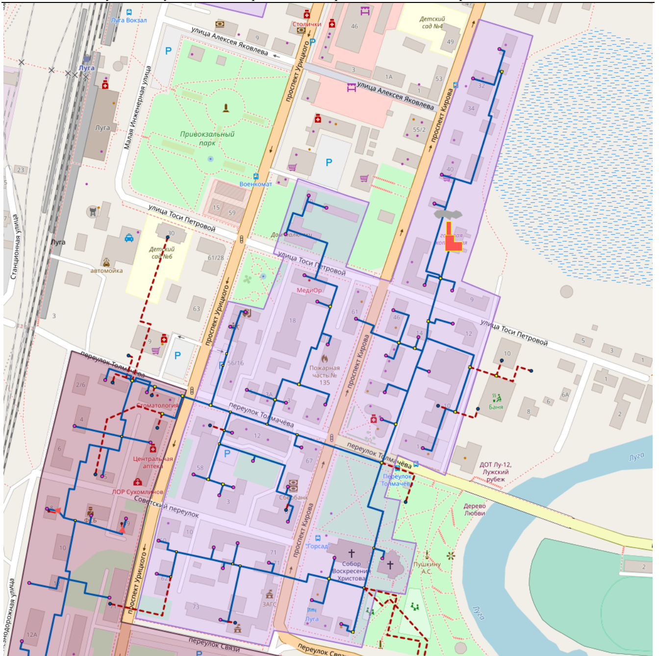
Рисунок 45 Зона действия котельной БМК-12,8 (ООО «Петербургтеплоэнерго»)
