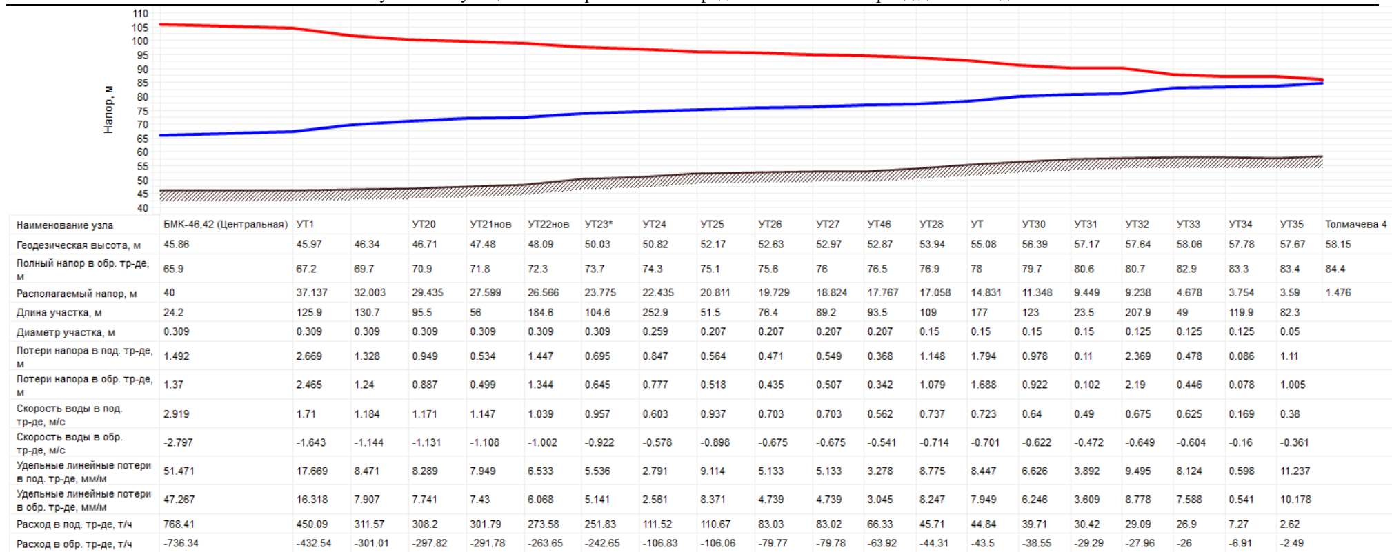
Рисунок 30 Пьезометрический график котельной БМК -46,42 (ООО «Петербургтеплоэнерго»)
