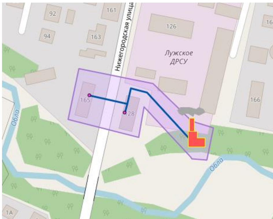
Рисунок 54 Зона действия котельной ул. Нижегородская (ООО «ТК Северная»)
