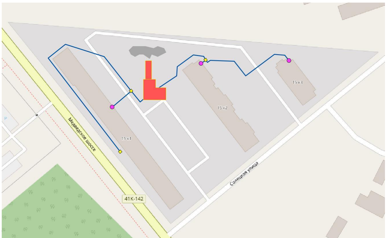
Рисунок 23 Тепловые сети котельной ООО «Спецзастройщик ЛО 1»
