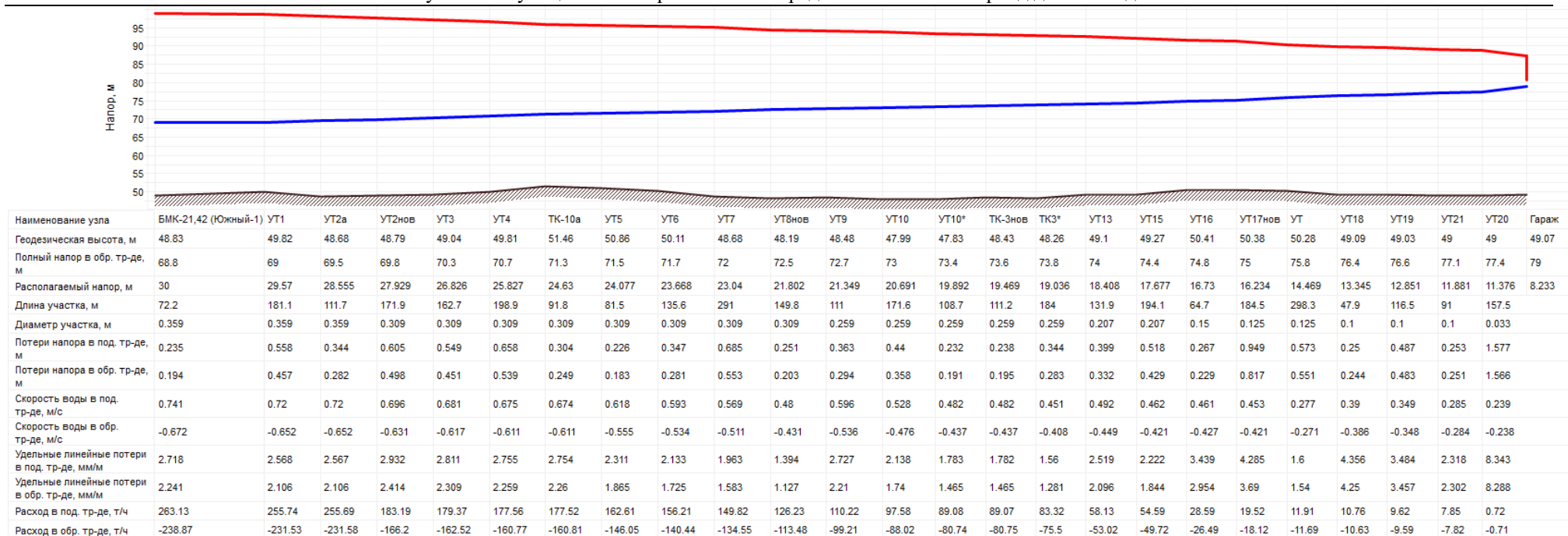
Рисунок 38 Пьезометрический график котельной БМК -21,42, Южный-1 (ООО «Петербургтеплоэнерго»)
