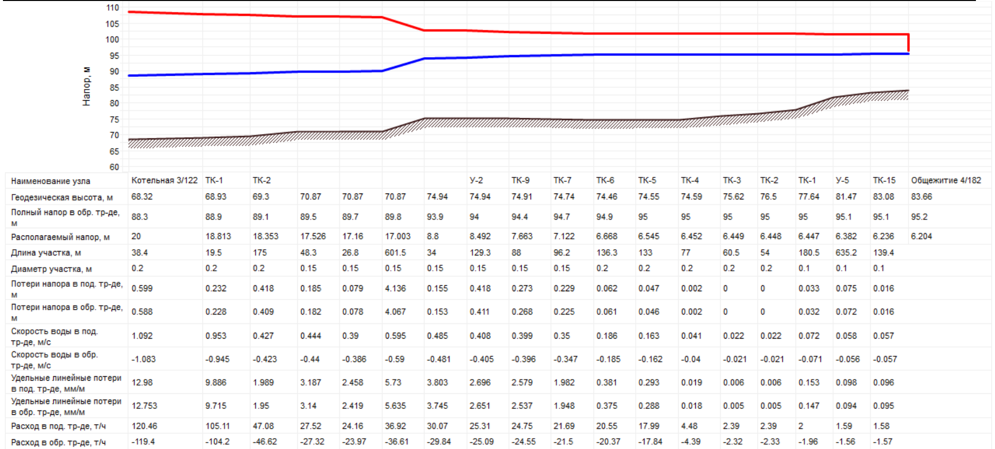
Рисунок 33 Пьезометрический график котельной №3/122 (ООО «Теплострой Плюс»)
