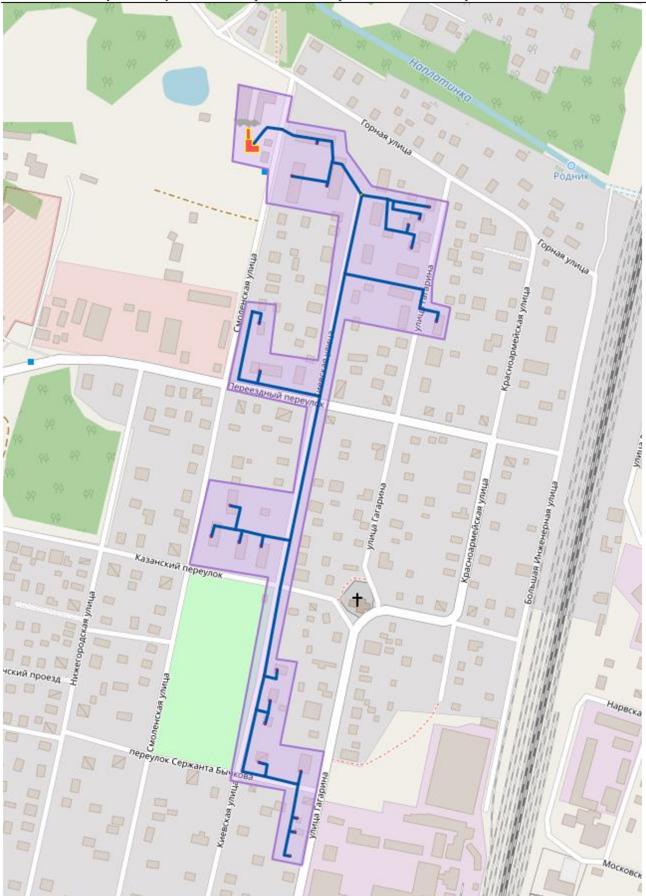
Рисунок 59 Зона действия котельной ул. Смоленская (ООО «ТК Северная»)
