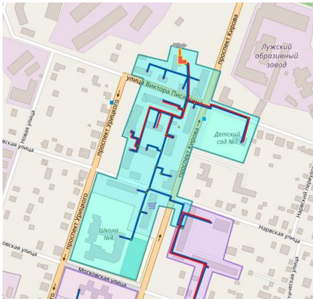
Рисунок 57 Зона действия котельной «Северная» (ООО «Тепловые системы»)
