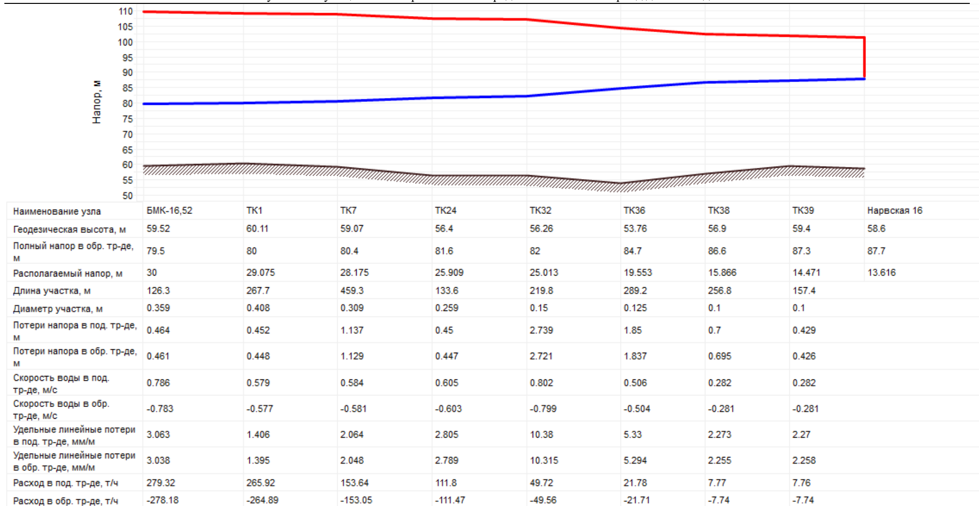
Рисунок 29 Пьезометрический график котельной БМК -16,52 (ООО «Петербургтеплоэнерго»)
