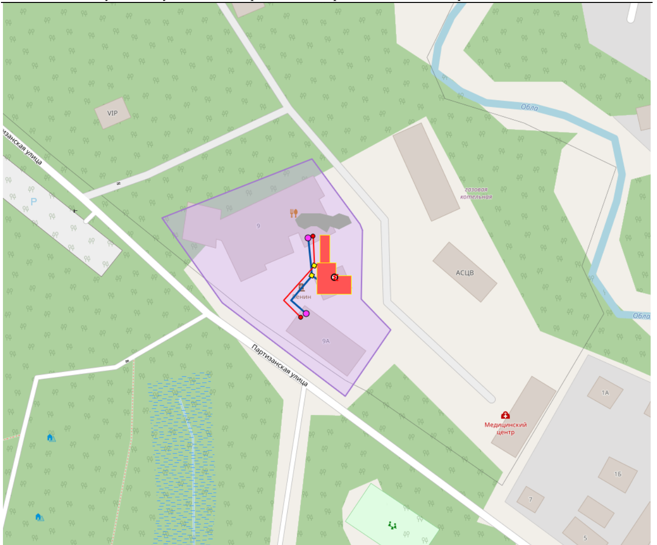
Рисунок 52 Зона действия котельной «Буревестник» (ГУП «Водоканал Санкт-Петербурга»)
