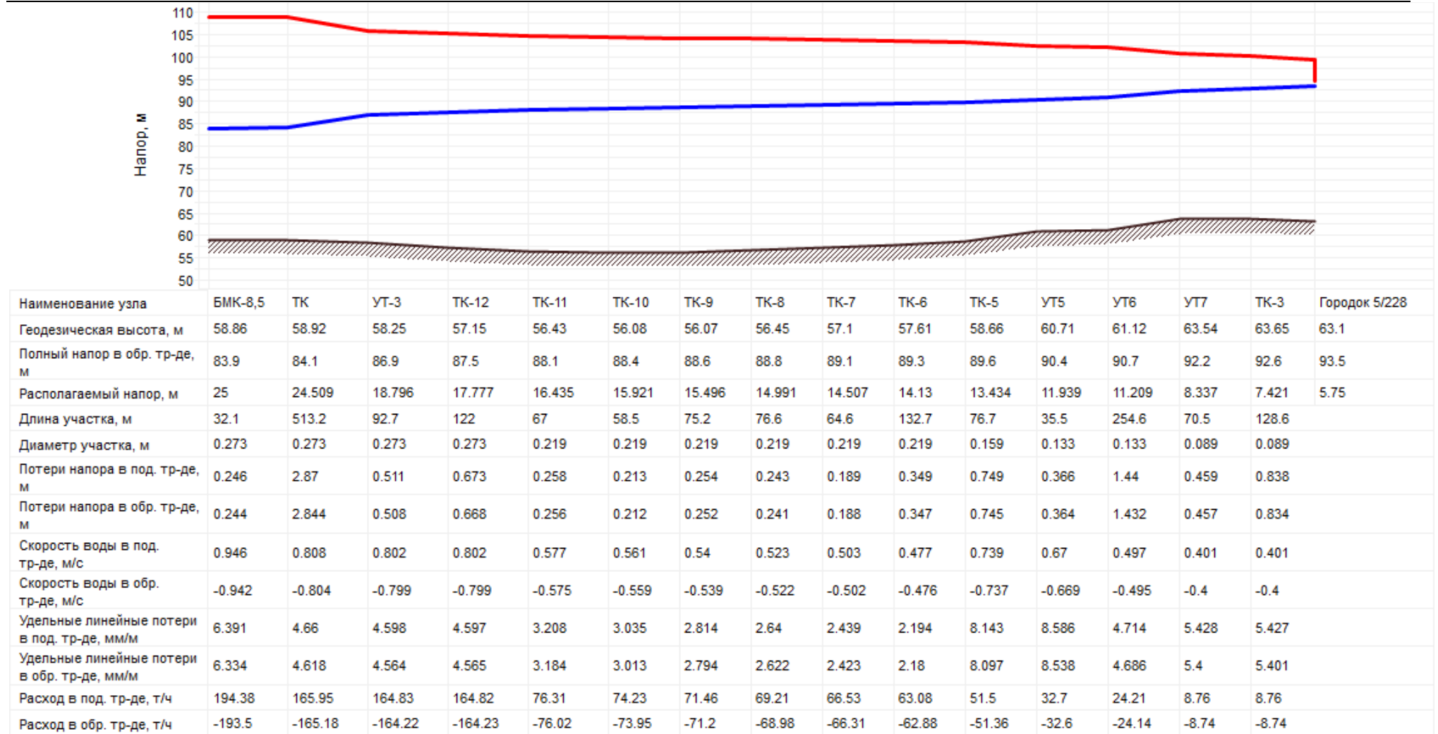
Рисунок 27 Пьезометрический график котельной БМК -8,5 (ООО «Петербургтеплоэнерго»)
