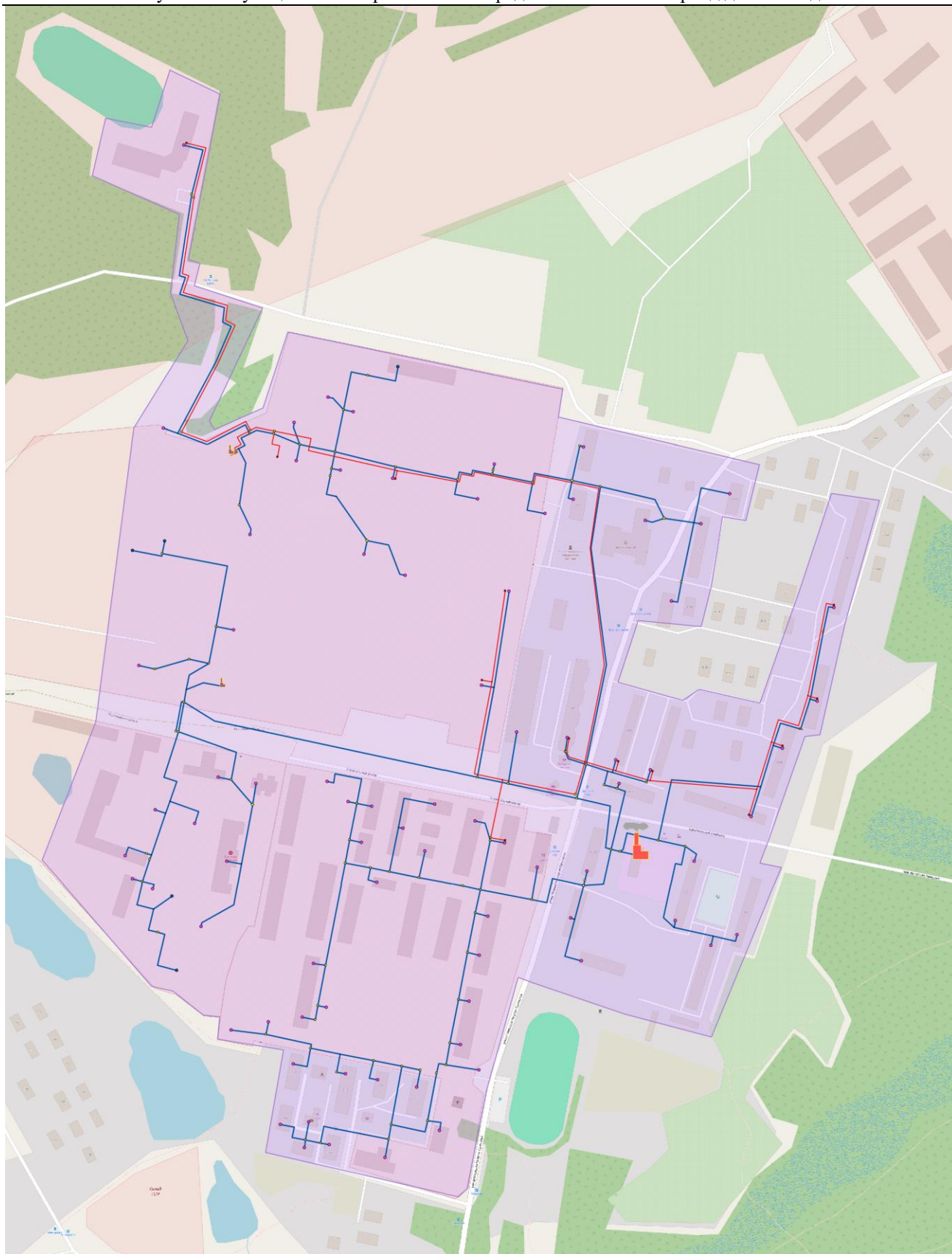
Рисунок 50 Зона действия котельной №3/122 (ООО «Теплострой Плюс»)
