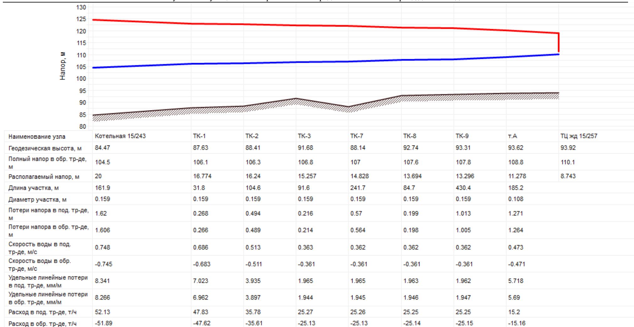
Рисунок 34 Пьезометрический график котельной №15/243 (ООО «Теплострой Плюс»)
