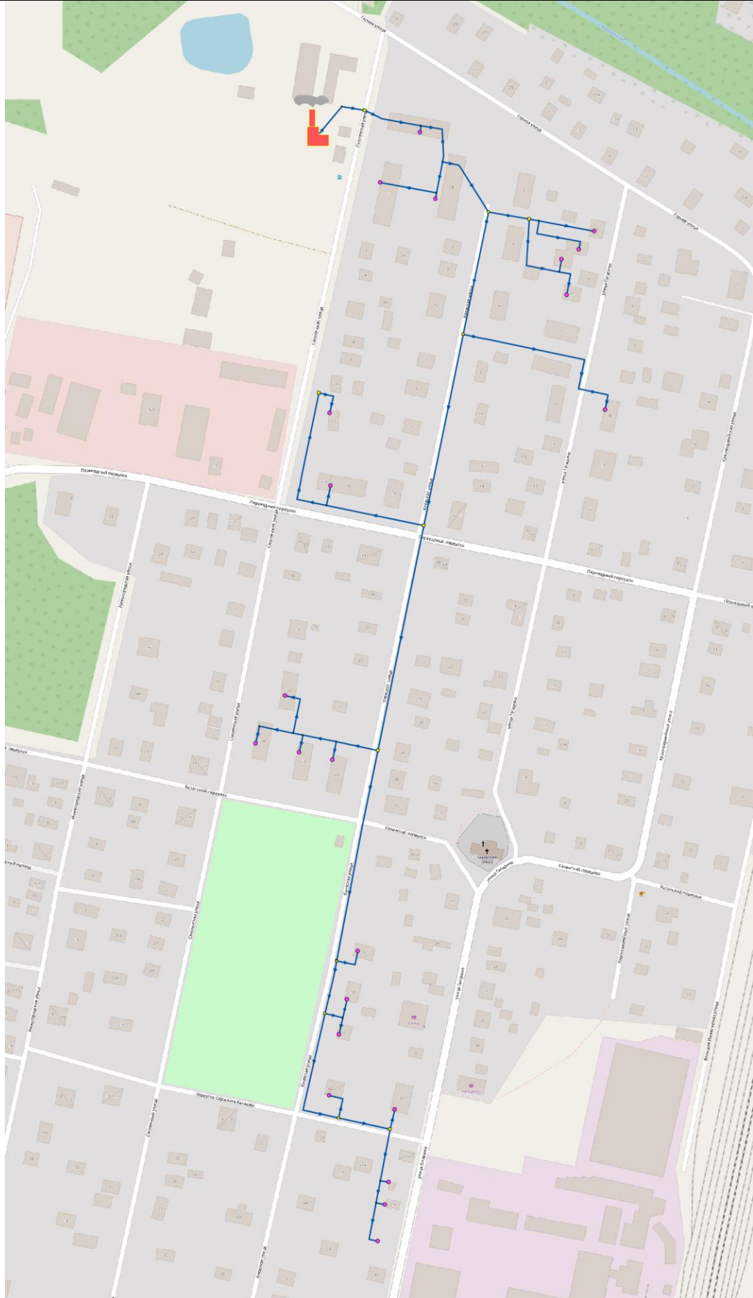
Рисунок 63 Расположение перспективной котельной по ул. Смоленская, д.1
