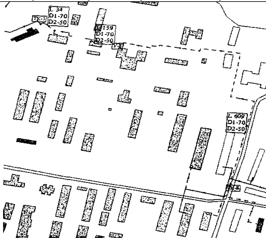
Рисунок 66 Схема прокладываемых и перекладываемых участков объединенной тепловой сети системы ГВС после осуществления второго этапа реконструкции
