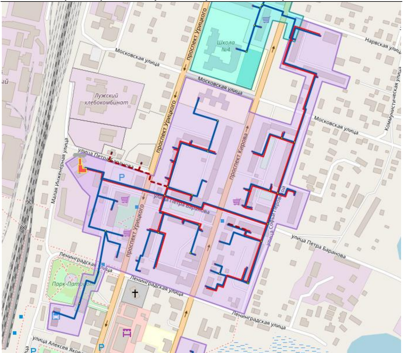
Рисунок 46 Зона действия котельной БМК-16,52 (ООО «Петербургтеплоэнерго»)
