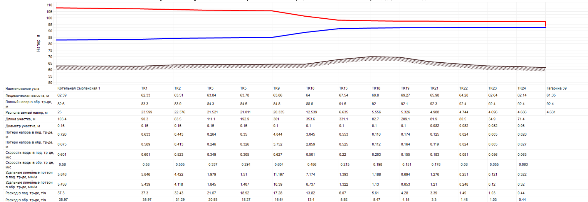
Рисунок 37 Пьезометрический график котельной ул. Смоленская (ООО «ТК Северная»)
