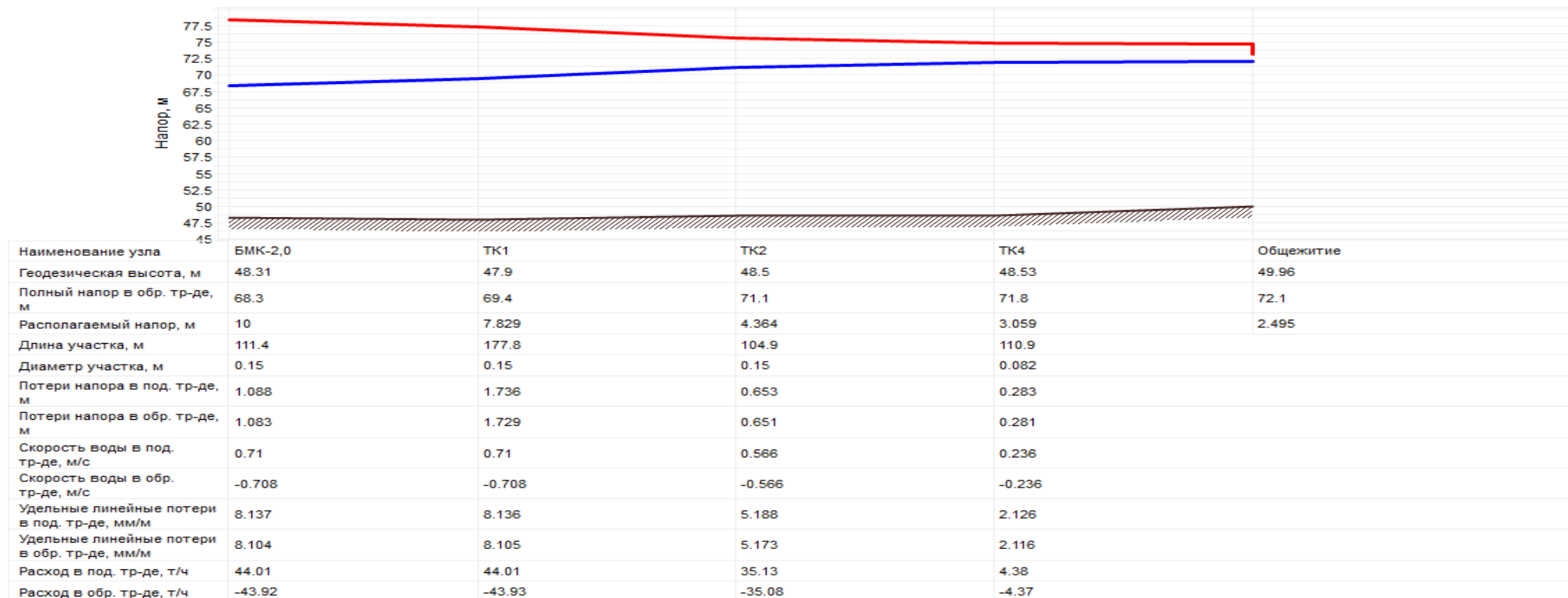
Рисунок 24 Пьезометрический график котельной БМК -2,0 (ООО «Петербургтеплоэнерго»)
