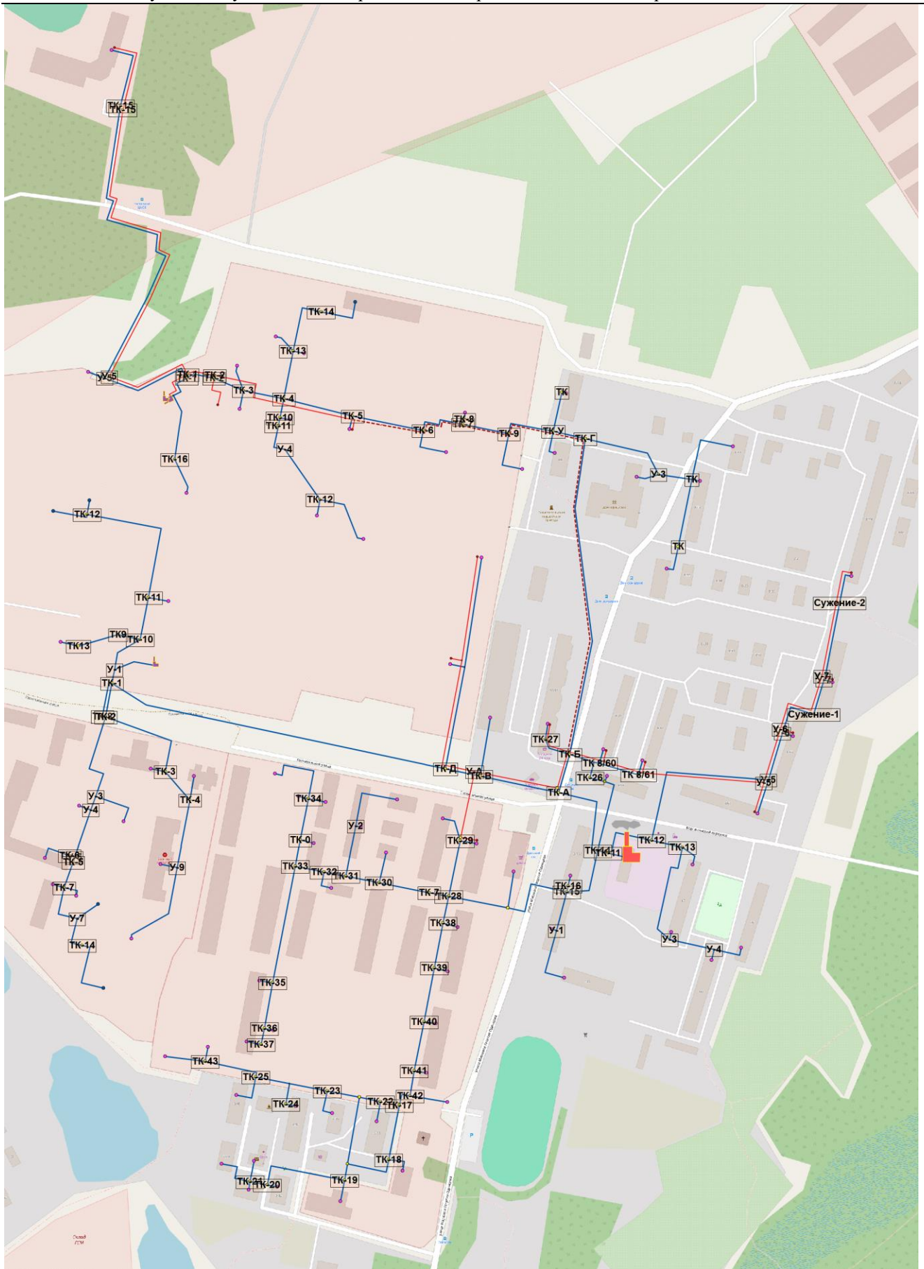
Рисунок 18 Тепловые сети котельных №3/122, и №4/180
