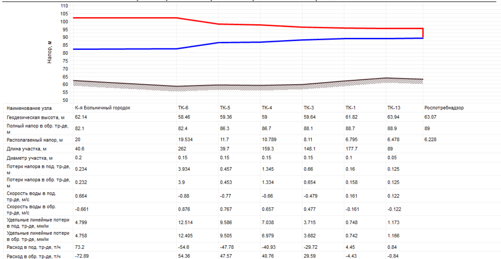
Рисунок 31 Пьезометрический график котельной Больничный городок (ООО «Лентепло»)
