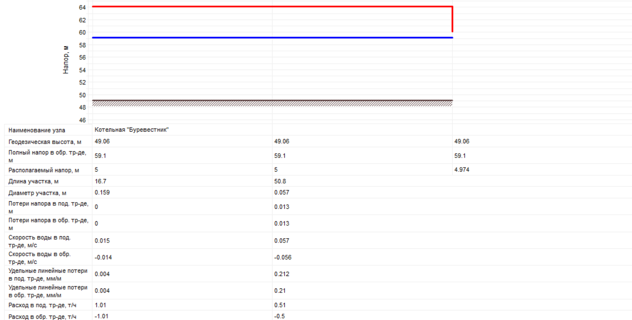
Рисунок 32 Пьезометрический график котельной Буравестник (ГУП «Водоканал Санкт-Петербурга»)
