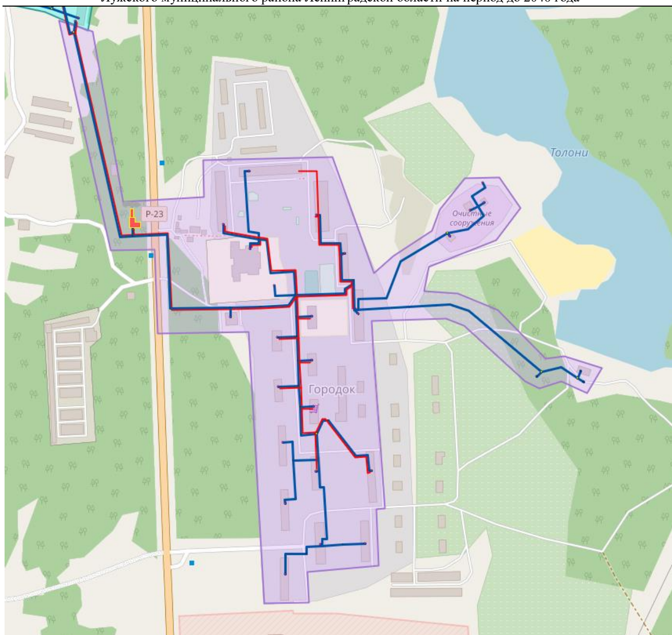
Рисунок 44 Зона действия котельной БМК-8,5 (ООО «Петербургтеплоэнерго»)
