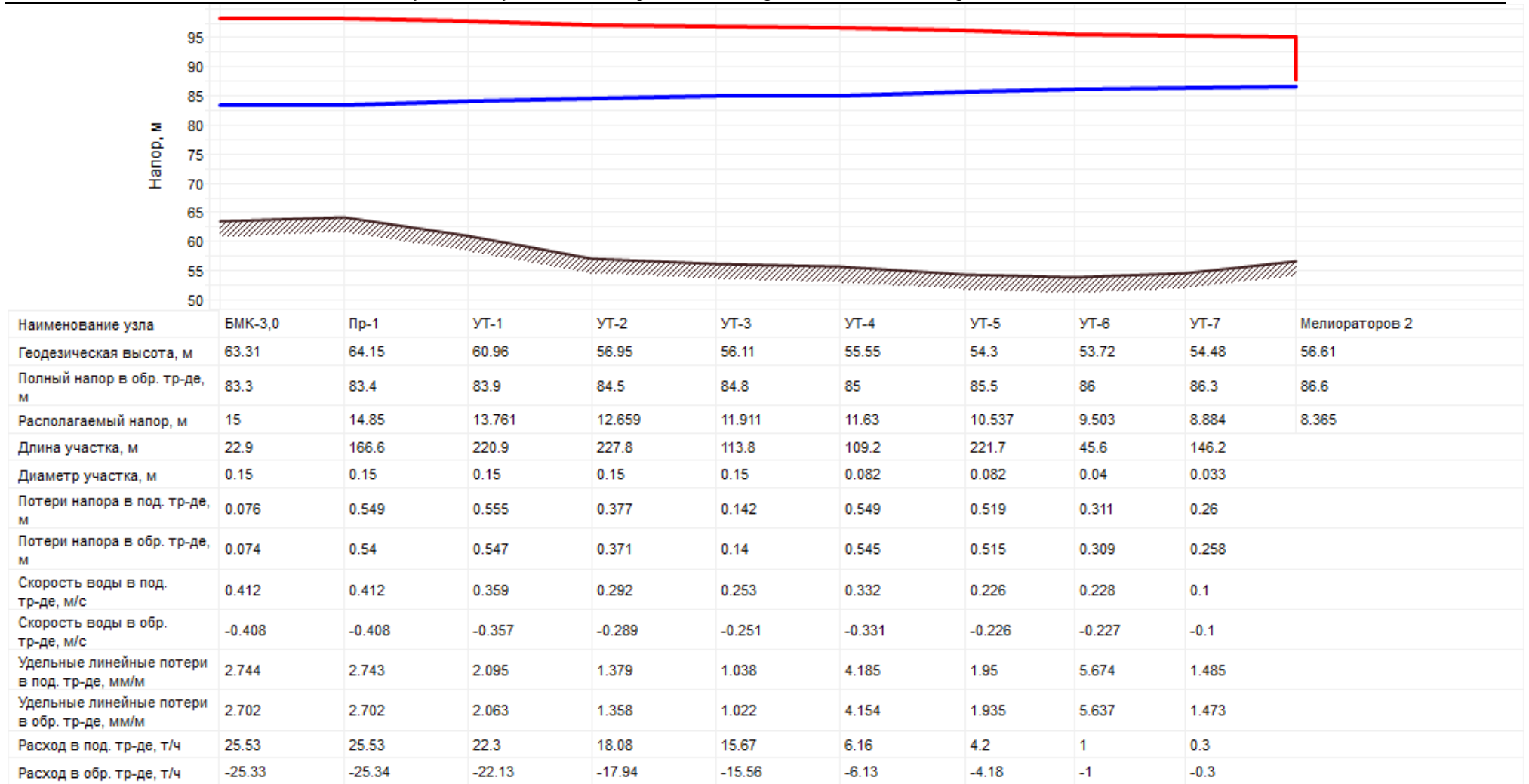
Рисунок 25 Пьезометрический график котельной БМК -3,0 (ООО «Петербургтеплоэнерго»)
