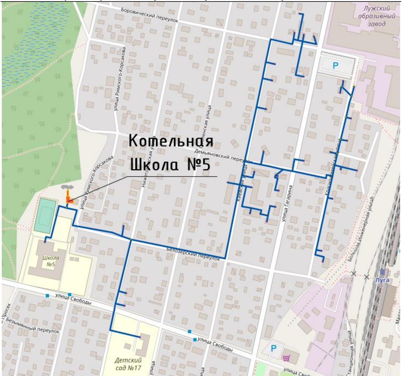
Рисунок 21 Тепловые сети котельной «Школа №5» (ул. Свободы)
