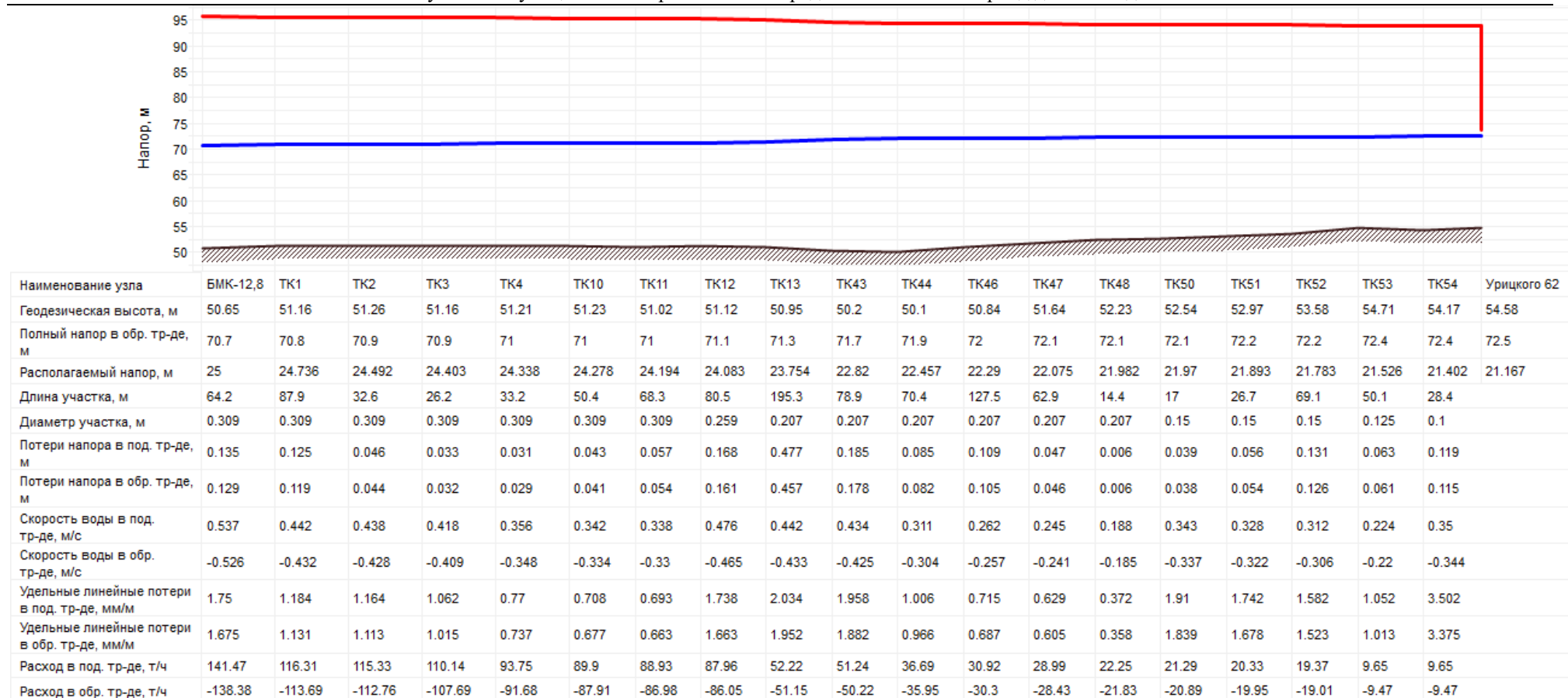
Рисунок 28 Пьезометрический график котельной БМК -12,8 (ООО «Петербургтеплоэнерго»)
