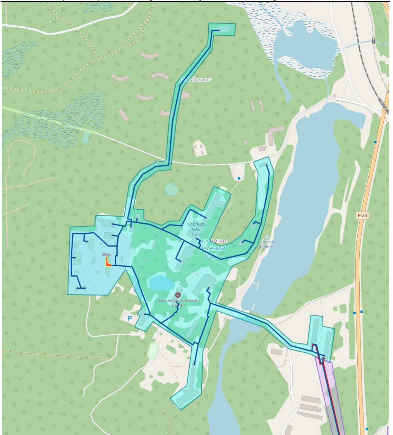
Рисунок 55 Зона действия котельной ООО «Зеленый Бор» (ОО «Зеленый Бор» ЦБ РФ)
