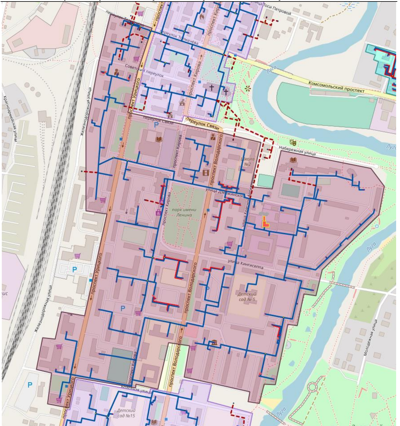
Рисунок 49 Зона действия котельной БМК-46,52, Центральная (ООО «Петербургтеплоэнерго»)
