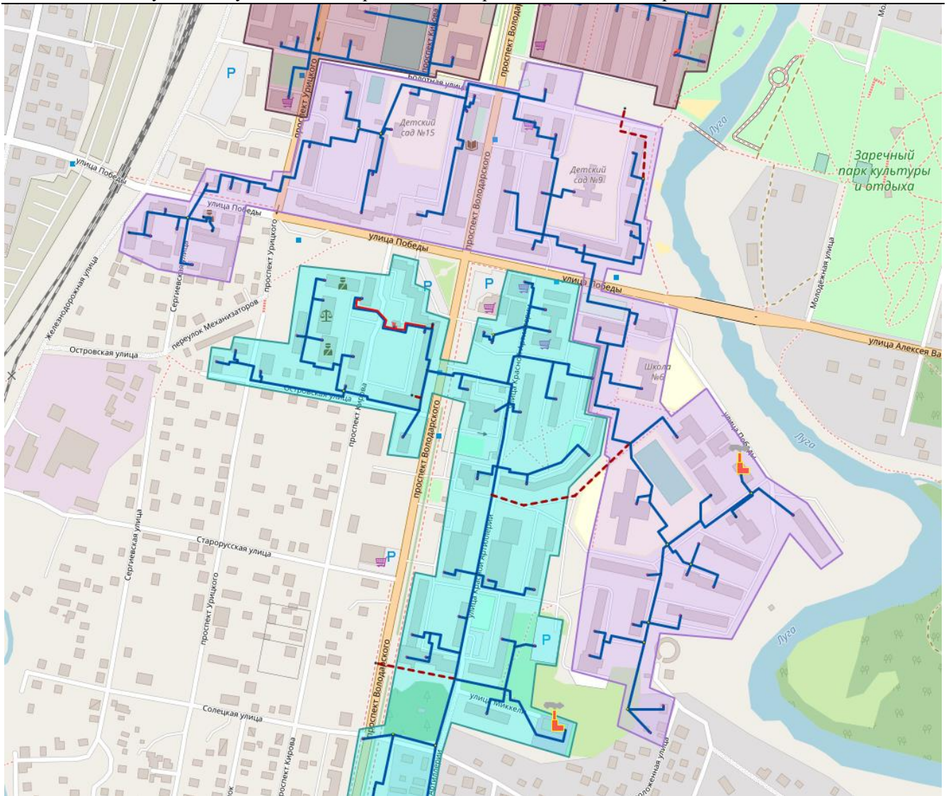
Рисунок 47 Зона действия котельной БМК-21,42, Южный-1 (ООО «Петербургтеплоэнерго»)
