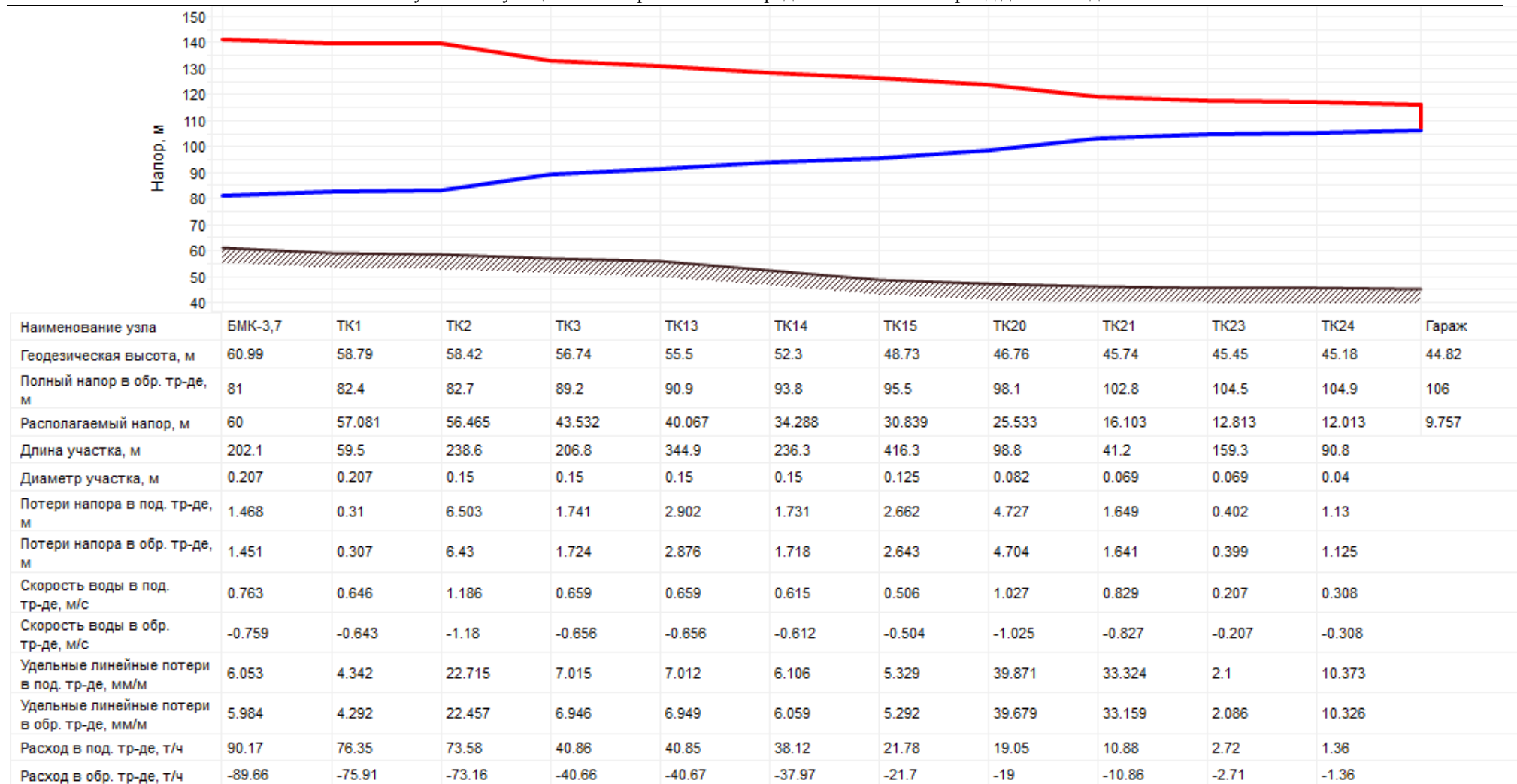
Рисунок 26 Пьезометрический график котельной БМК -3,7 (ООО «Петербургтеплоэнерго»)
