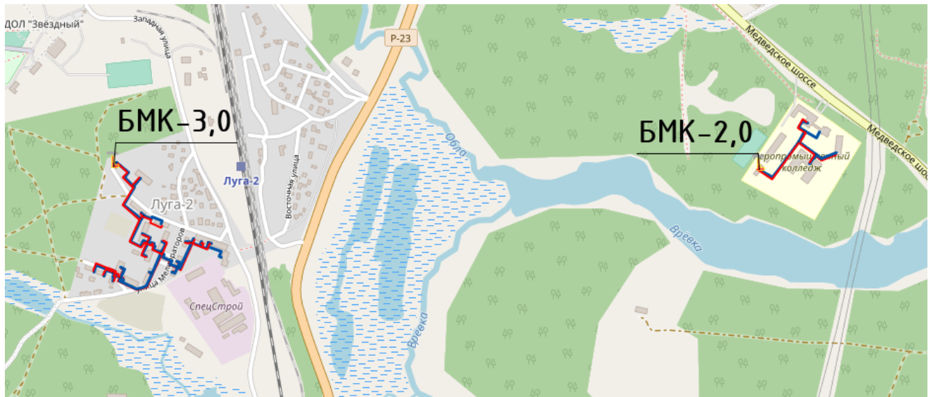
Рисунок 15 Тепловые сети котельных БМК-2,0 МВт и БМК-3,0 МВт
