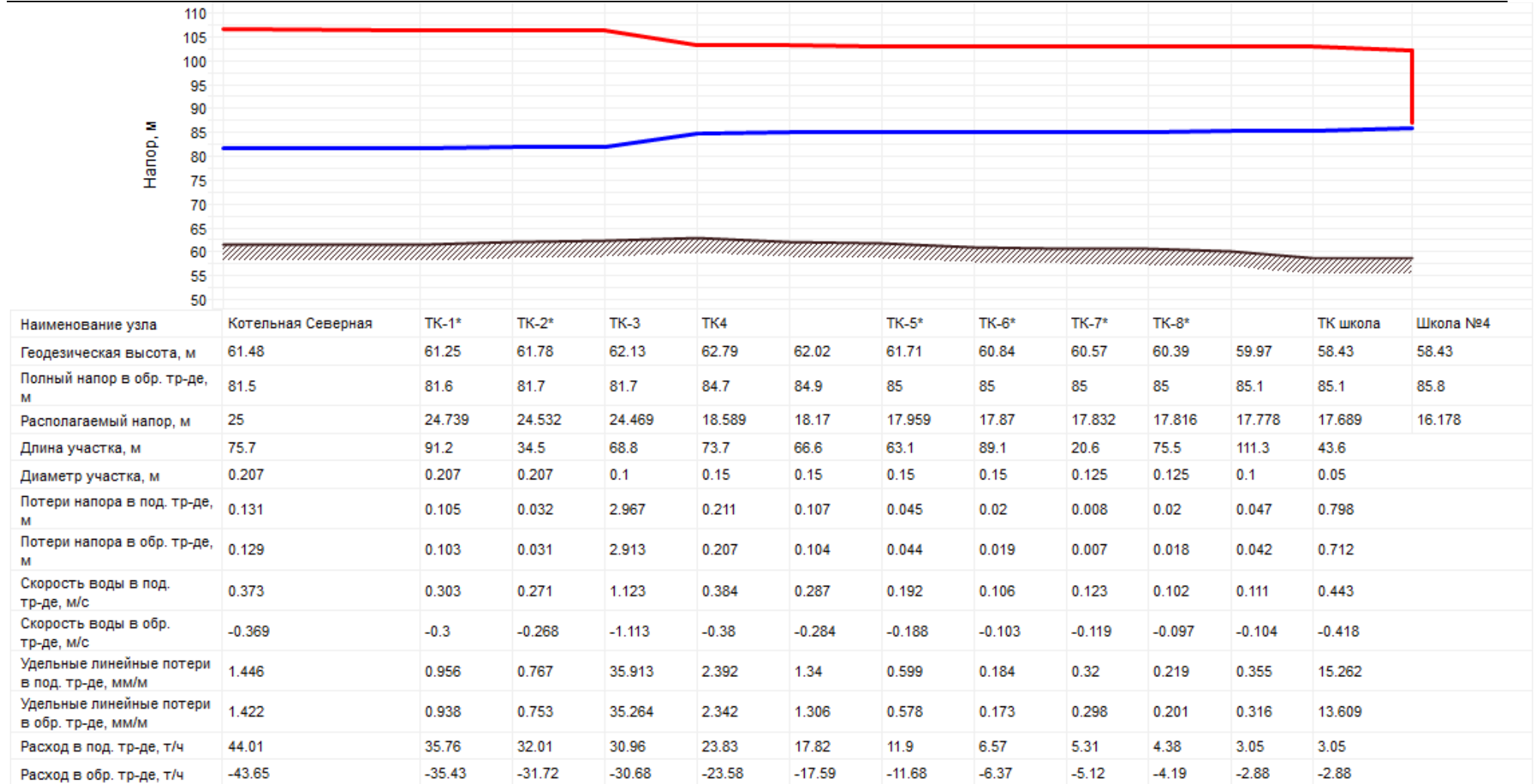
Рисунок 36 Пьезометрический график котельной «Северная» (ООО «Тепловые системы»)
