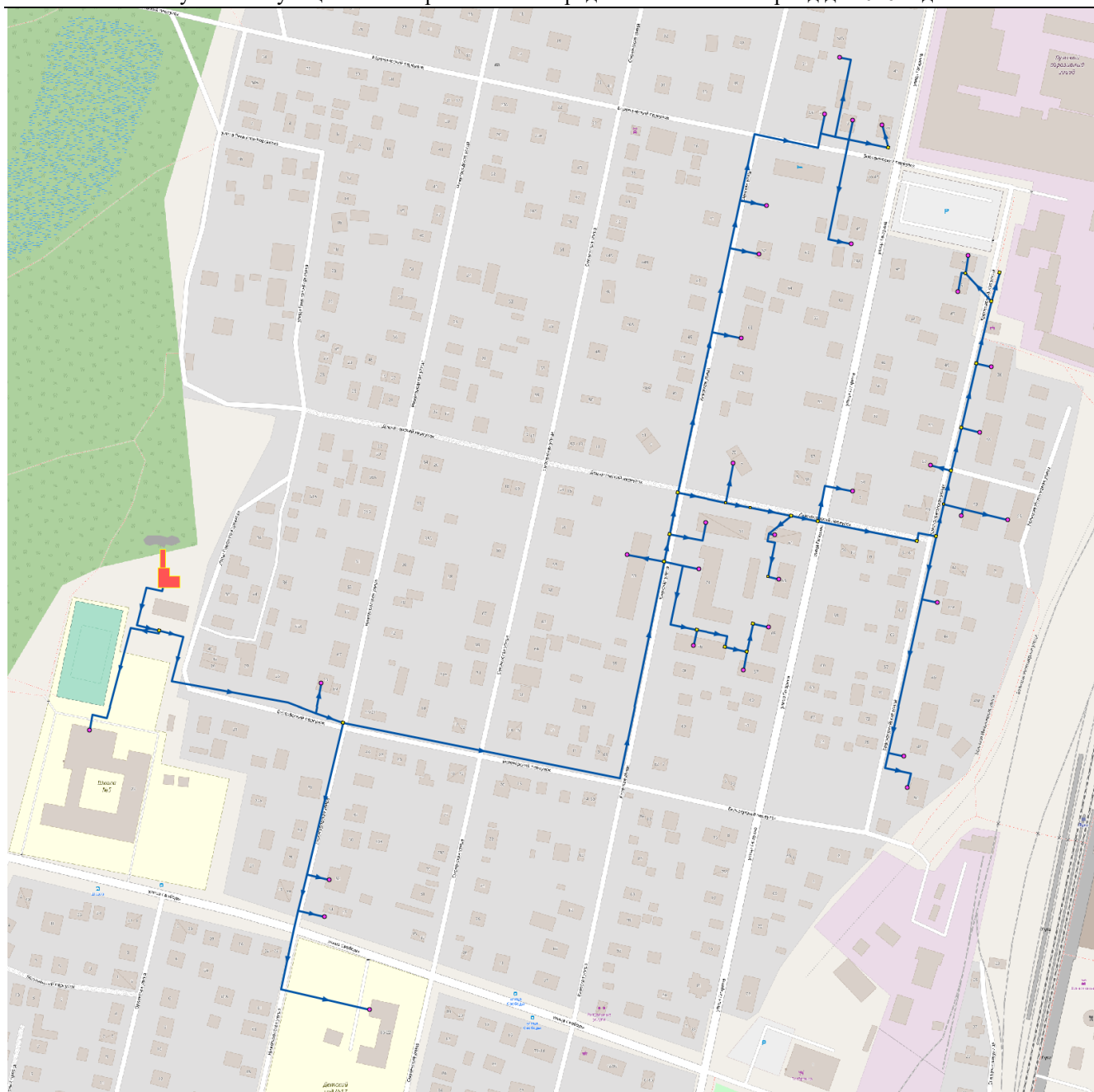
Рисунок 62 Расположение перспективной котельной по ул. Свободы, д.23
